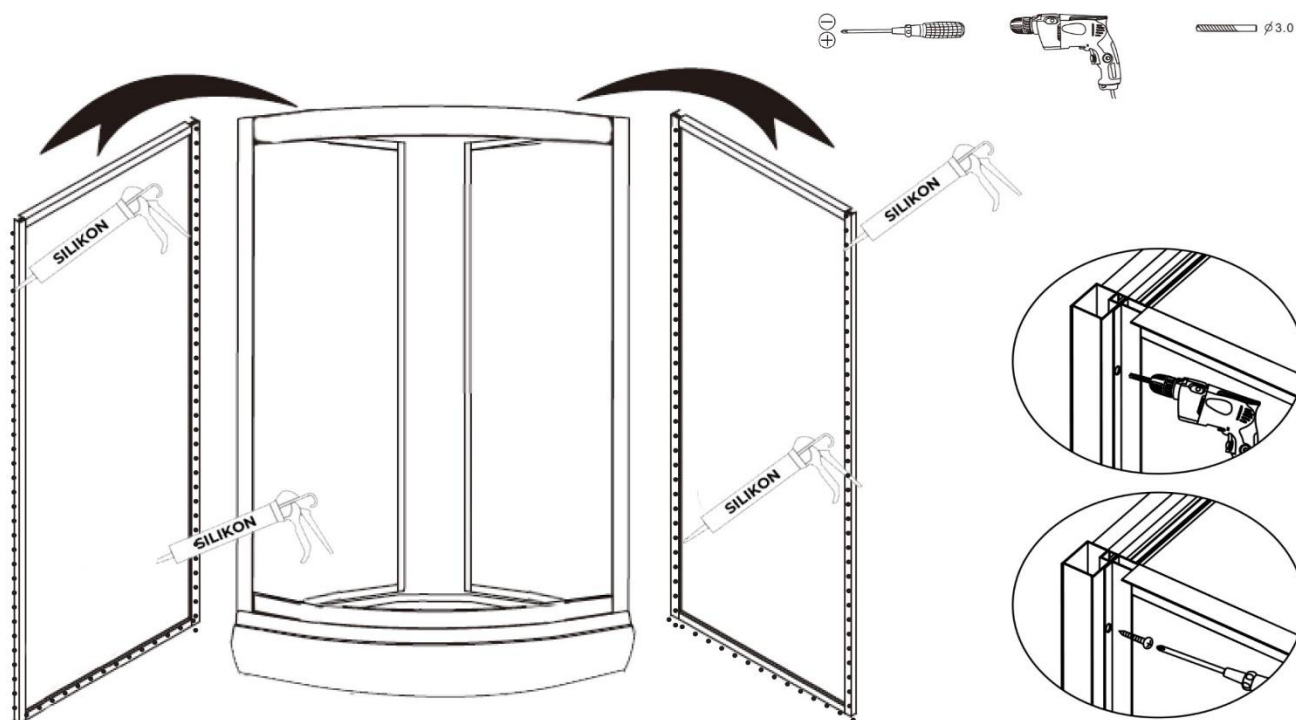
Přišroubování zadní stěny k přednímu profilu.
