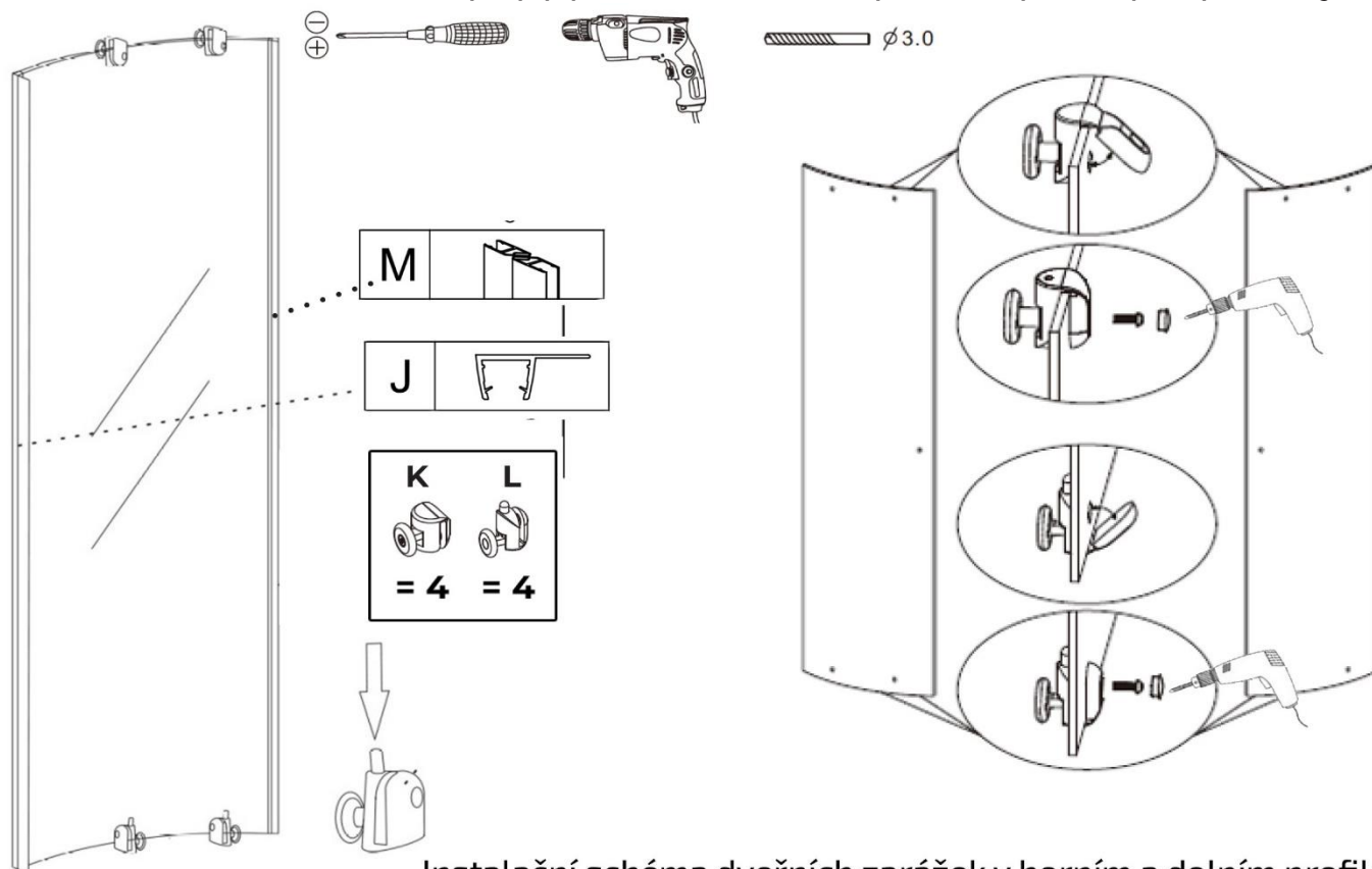
Instalační schéma dveřních zarážek v horním a dolním profilu.
