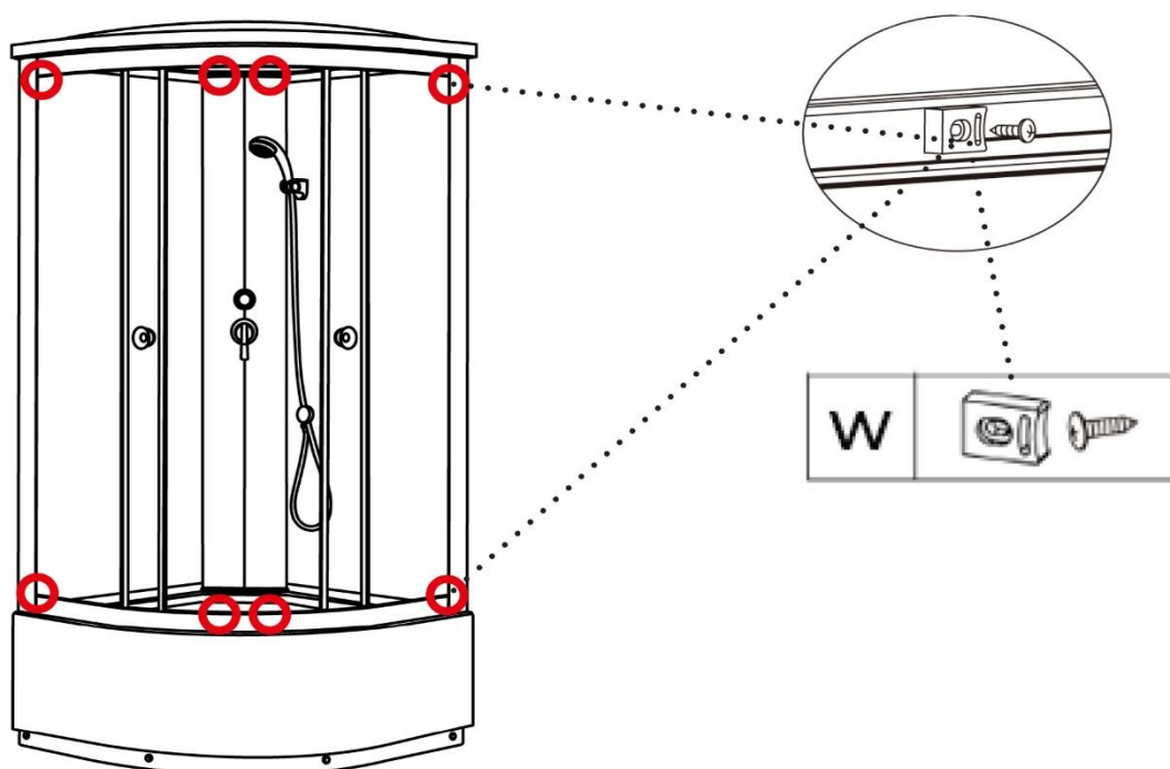
Instalační schéma dveřních zarážek v horním a dolním profilu.
