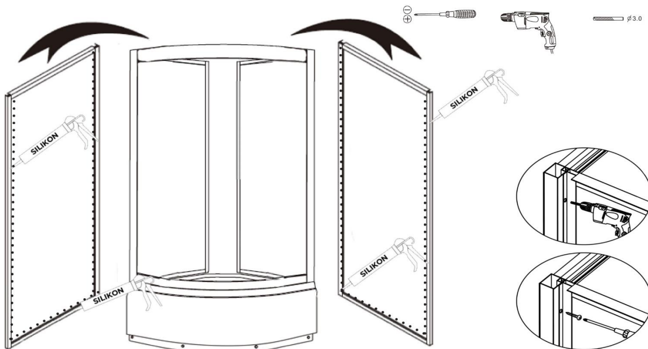
Přišroubování zadních stěn do předního profilu.
