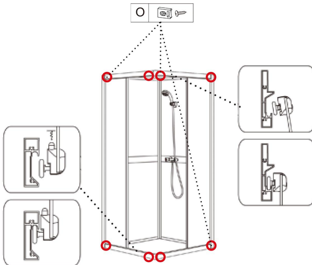
Montáž dveřních zámků do horního a dolního profilu rámu kabiny.
