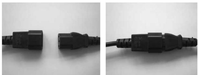
Způsob připojení topných panelů
